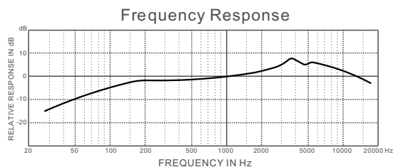
Snare 典型频率响应 (图6)
