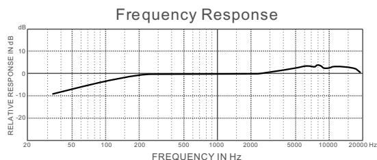
E102 典型频率响应 (图8)
