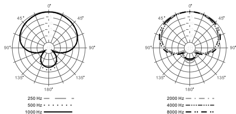
E102 典型的超心型极坐标图型 (图7)
