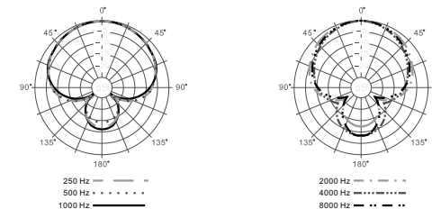
PRA218B 典型的超心型极坐标图型 (图1)
