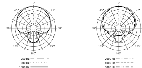
Tom tom 典型的超心型极坐标图型 (图3)
