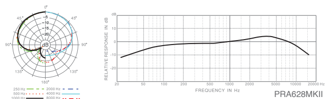
PRA628MKII 频率响应图 (超心型)
