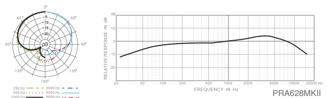
PRA628MKII 頻率響應圖 (超心型)
