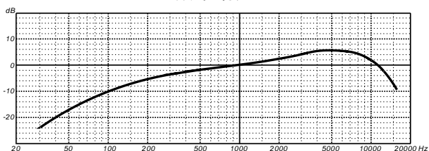
频率响应
