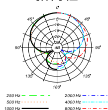
指向性
