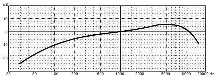
频率响应
