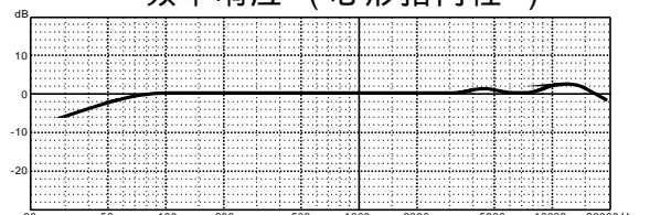
频率响应 (心形指向性)
