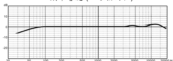
頻率響應(心形指向性)
