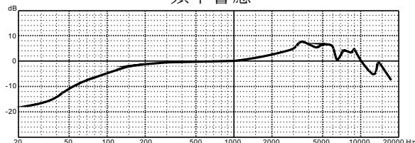
頻率響應
