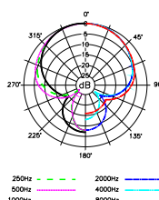
指向性
