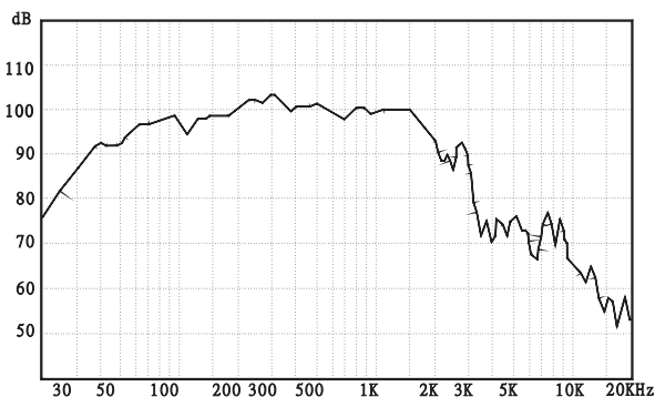
頻響曲線圖
