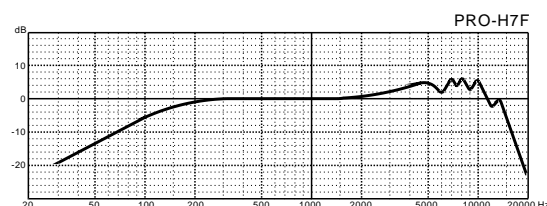
频率响应
