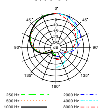
指向性
