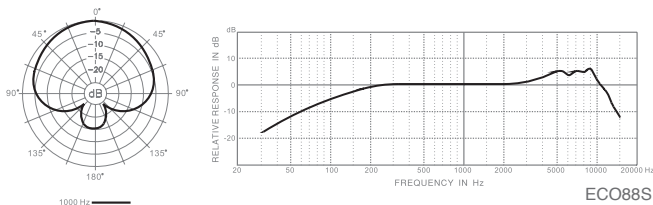
EC088S 頻率響應圖（超心型）
