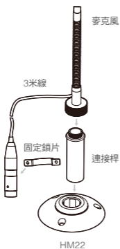
連結方法一
