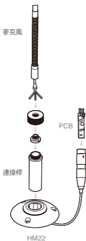
連結方法三
