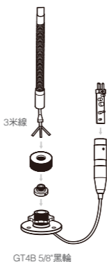
連結方法四
