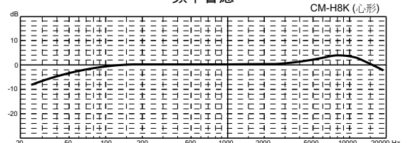
頻率響應
