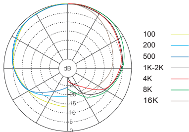
S502MKII频率响应图 (心型)
