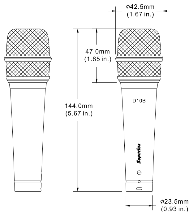
外型尺寸圖(圖3)
