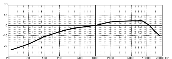
頻率響應
