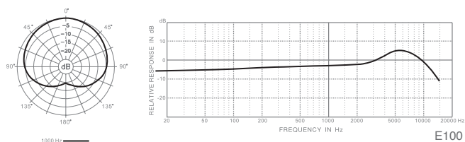
E100 频率响应图 (心型)
