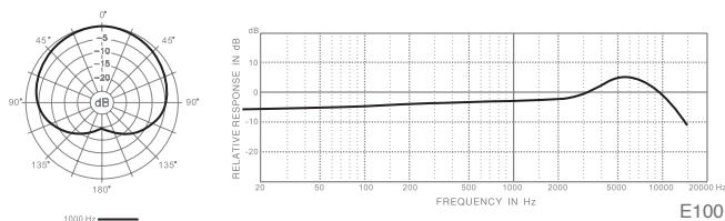
E100 頻率響應圖（心型）
