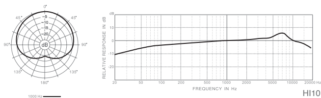
HI10 频率响应图 (心型)
