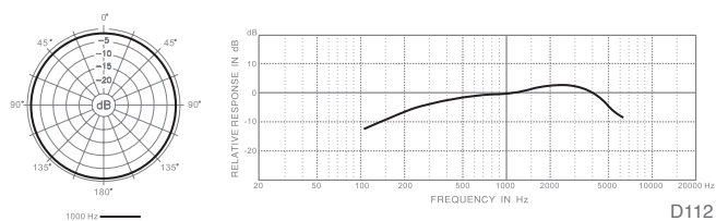
D112C 频率响应图（无指向）
