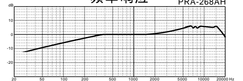
频率响应 PRA-268AH
