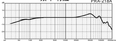
频率响应 PRA-218A
