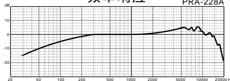
频率响应 PRA-228A
