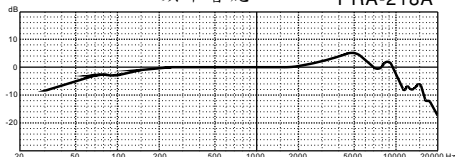
頻率響應 PRA-218A
