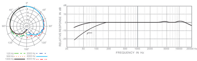
L211 频率响应图（心型）
