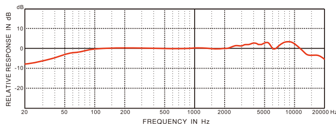
D108MKII 頻率響應圖（超心型）
