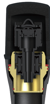
D108MKII 剖面圖
