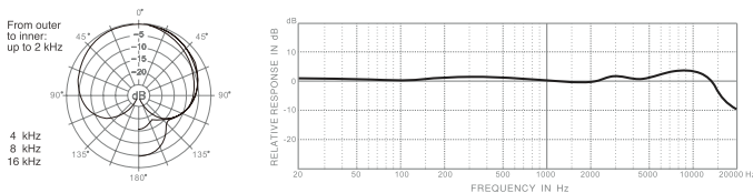
S502 頻率響應圖（心型）
