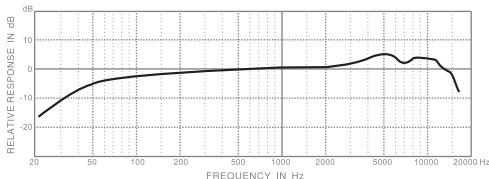
PRO228A
